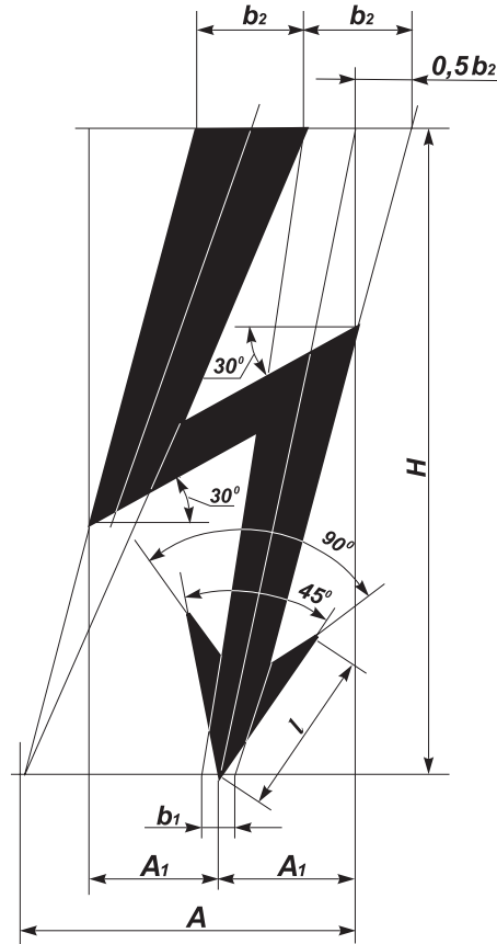
Рисунок Л.1 – Графический символ электрического напряжения
